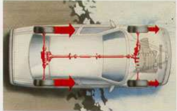
Das Prinzip der Ferguson Visco-Kupplung
