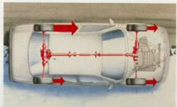
Hinterachse mit Torsen- Differential
